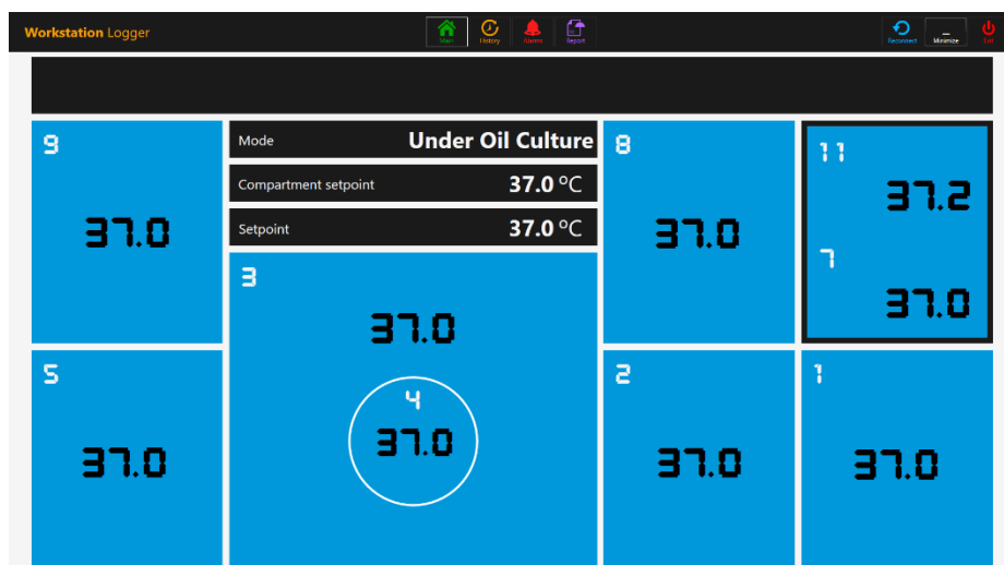
Figur 23.4 Vy av arbetsstationens loggning på den 2:a displayen under normala arbetsförhållanden (med en gasblandare)
