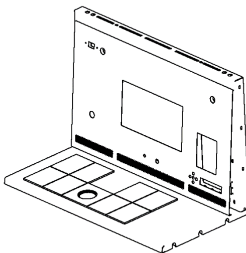
Figur 11.6 Multi-zone ART-arbetsstationen utan kammare
